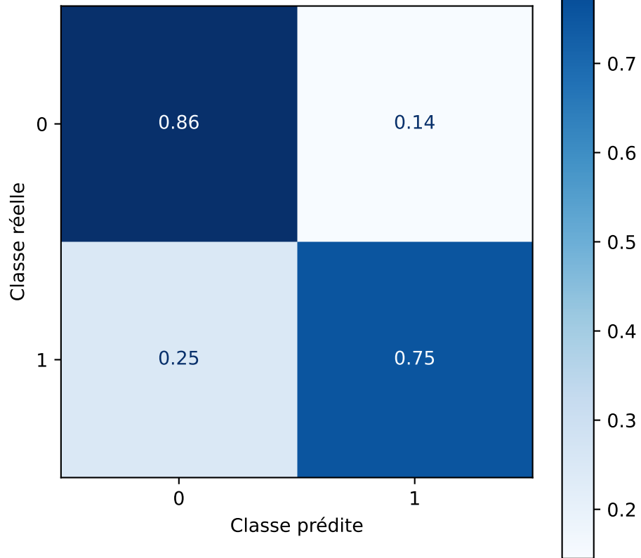
(b) Matrice de confusion normalisée
