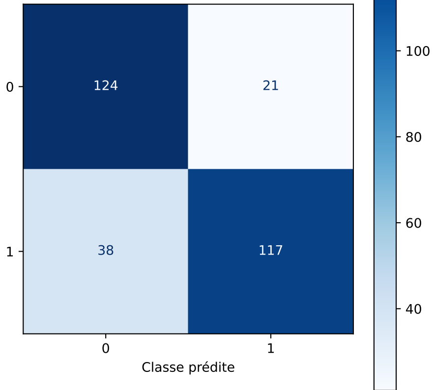
(a) Matrice de confusion non normalisée
